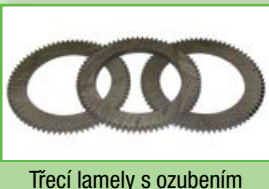
Třecí lamely s ozubením D420xD318x14-72Z FAG-M
